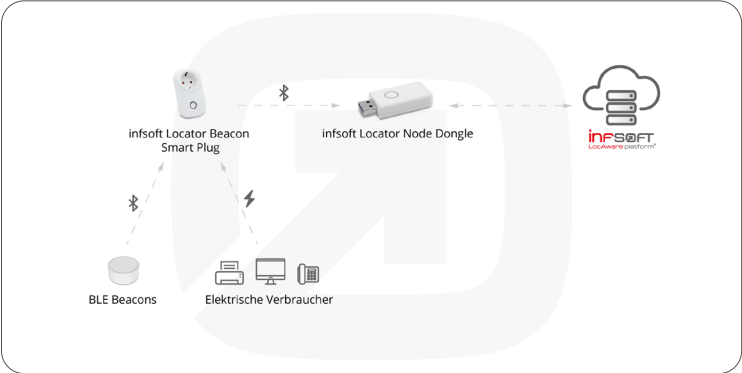
Energiemonitoring mit infsoft Locator Beacons Smart Plug
