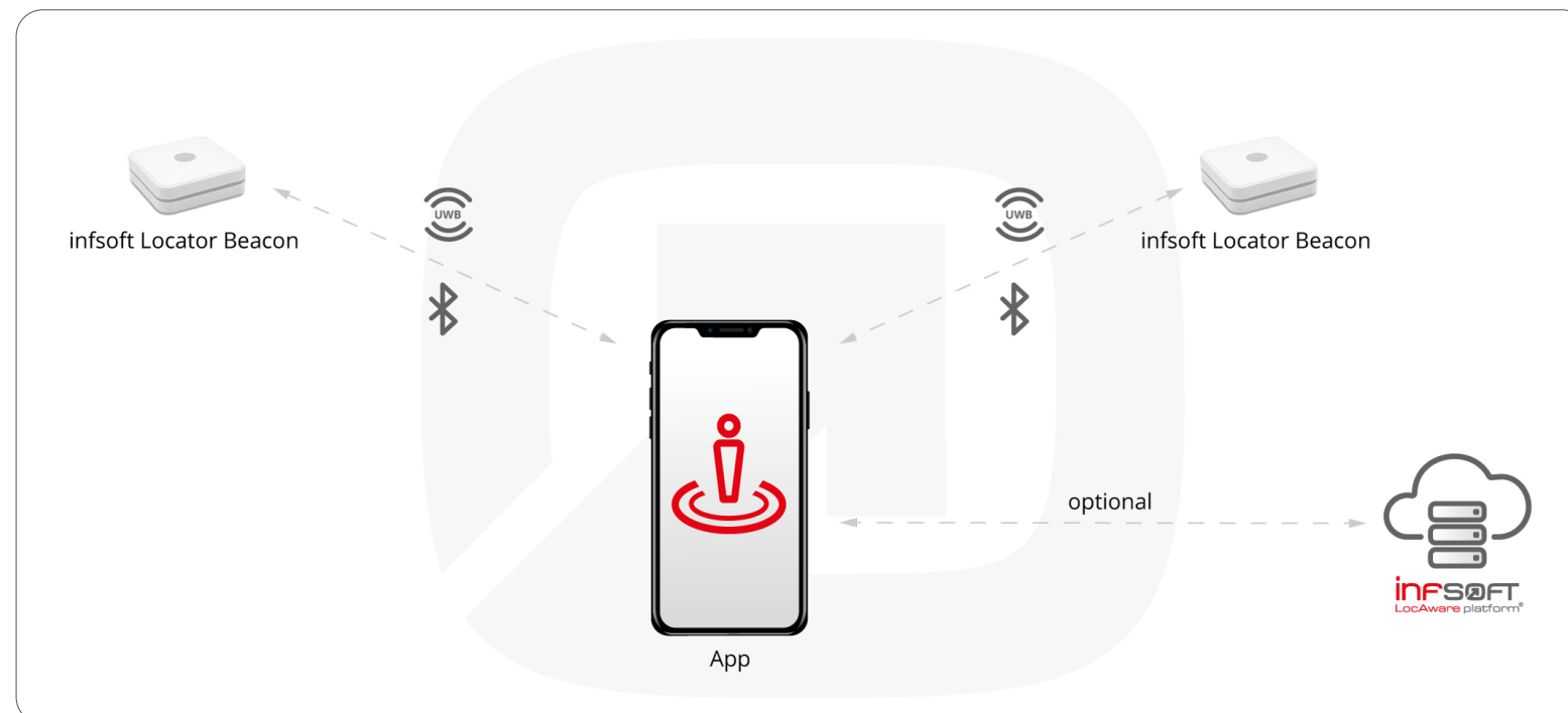
clientseitige Positionsbestimmung mit insoft Locator Beacons
