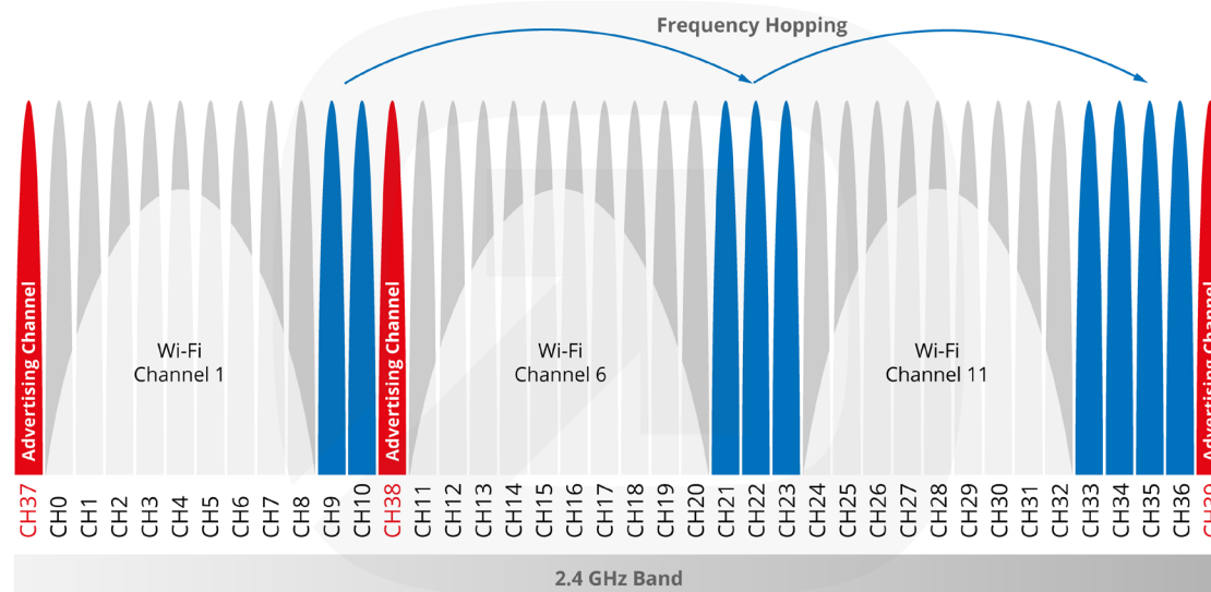
Optimale Nutzung der Funkkanäle bei der gleichzeitigen Verwendung von BLE und WLAN
