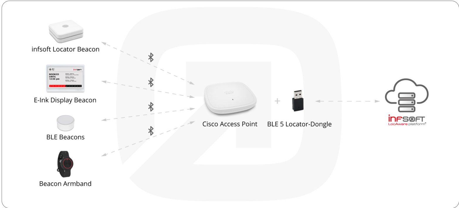
Nutzung von Cisco Access Points mit insoft Locator Node Firmware
