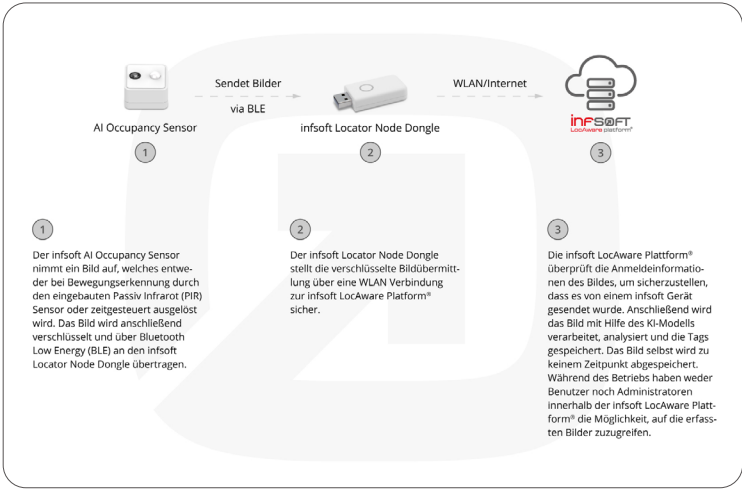
infsoft AI Occupancy Sensor Datenfluss
