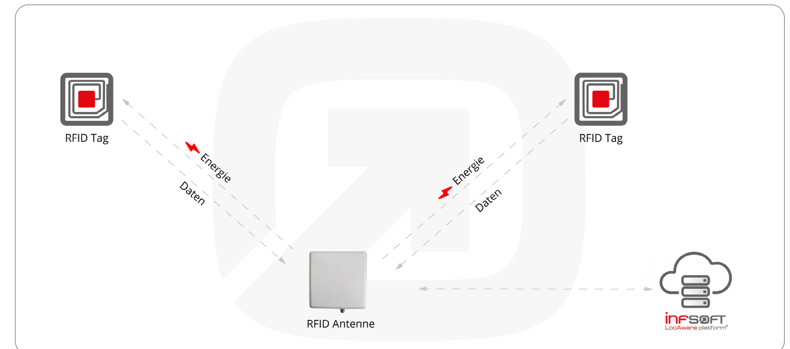
Kombination von RFID und UWB für die Identifikation und Verortung von Waren
